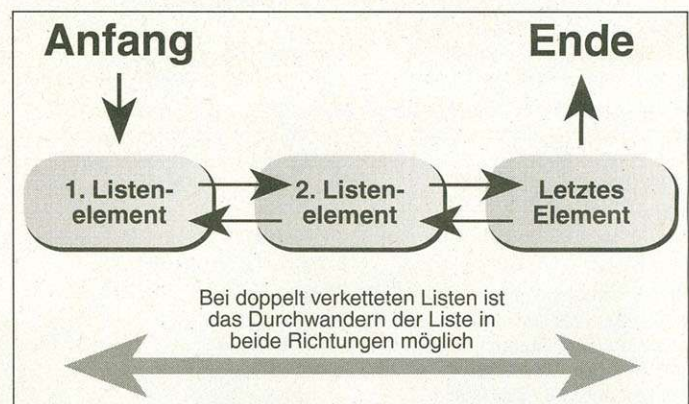
Doppelt verkettete Liste: Sie ermöglicht beliebiges Bewegen innerhalb der Liste und vereinfacht das Löschen
